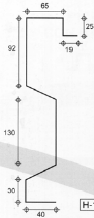
FALDON TRASERO CON PORTA LUZ INTEGRADO
