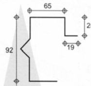
FALDON LATERAL
